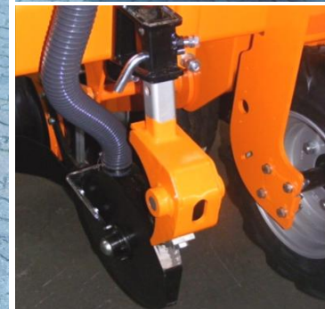
Asurcador a disco enganche rìgido (en versi3n con abonadora)
